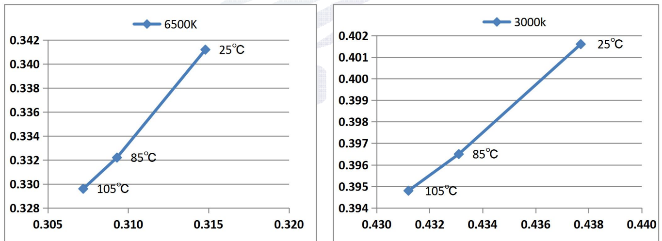
Fig 1-14 (x,y) Coordinates Vs Forward Current (x,y)坐标与正向电流特性曲线
