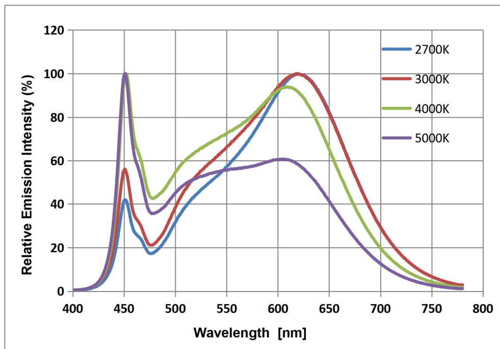
Fig 1-13 Spectrum Distribution 光譜分布特性曲線
