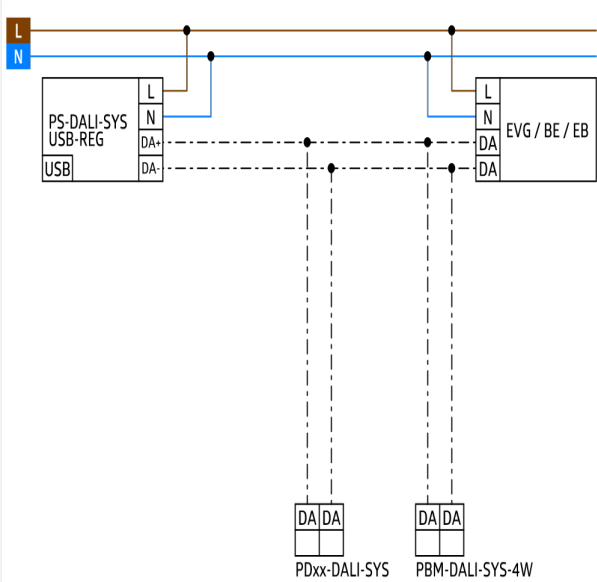
Wiring diagramms
