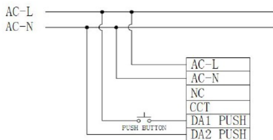
Diagrama de ligação para dimerização via PUSH
