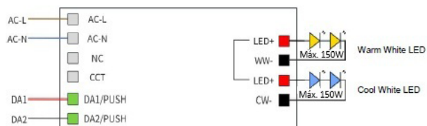
Saídas WW e CW conectadas a duas luminárias de cor única.
