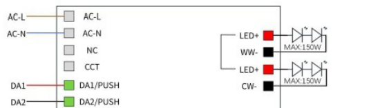
Saídas WW e CW conectadas a duas luminárias de cor única.
