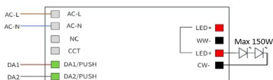
Saída CW conectada a uma luminária de cor única.
