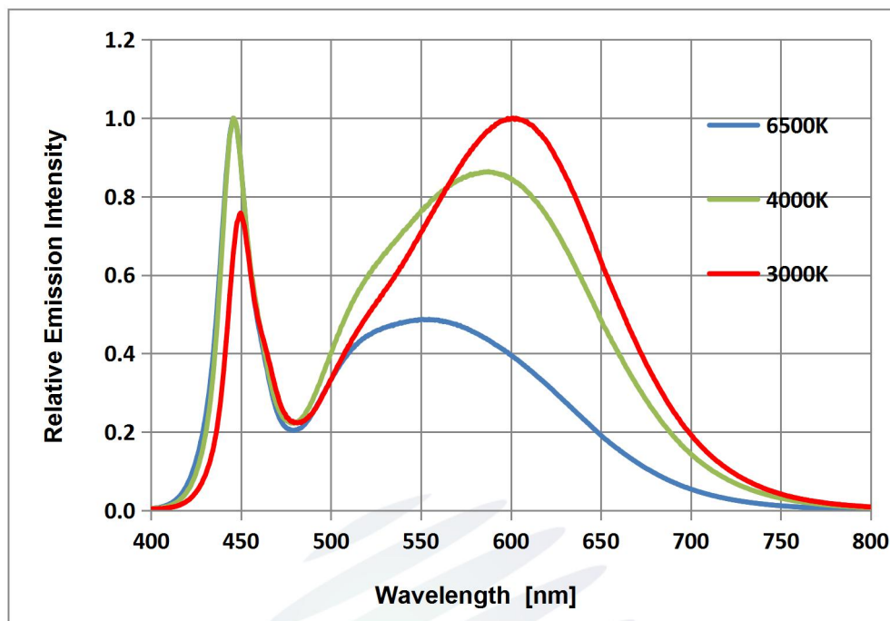
Fig 1-13 Spectrum Distribution光譜分布特性曲线
